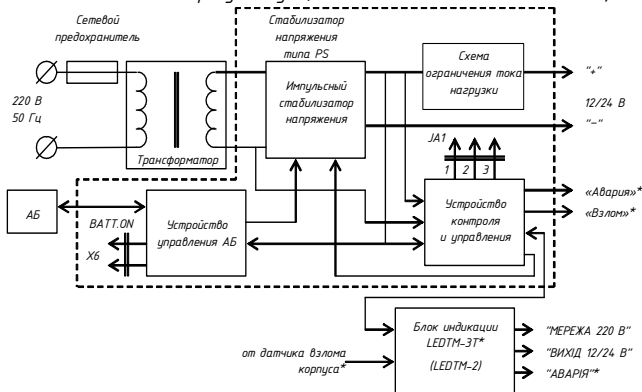
Рисунок 2. Схема источников бесперебойного электропитания тип PPS
