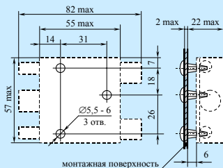
Распределитель VDR1x2R
